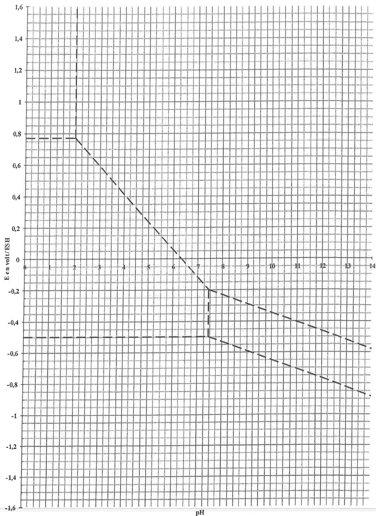
Diagramme potentiel pH de l'élément fer c = 0,01 \text{ mol.L}^{-1} , T = 298 \text{ K}
